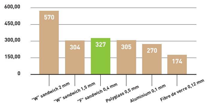
Graph 1 : Masse Surfacique en g / m 2
