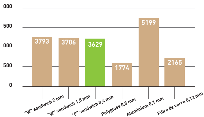
Graph 4 : Vitesse du son en m/s
