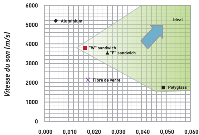
Graph 6 : Amortissement (tan delta)
