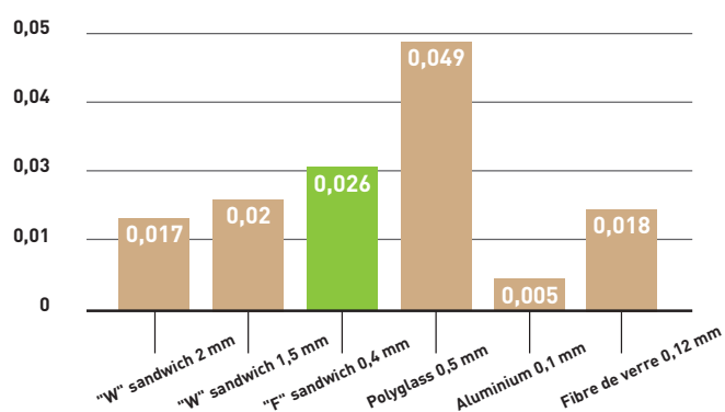
Graph 3 : Facteur de dissipation tan delta
