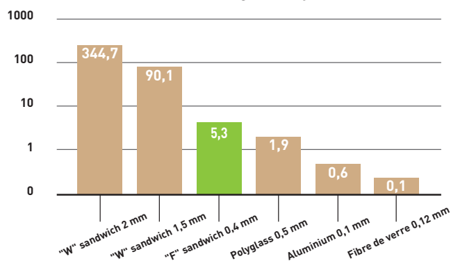
Graph 5 : Index de rigidité en flexion (échelle logarithmique)
