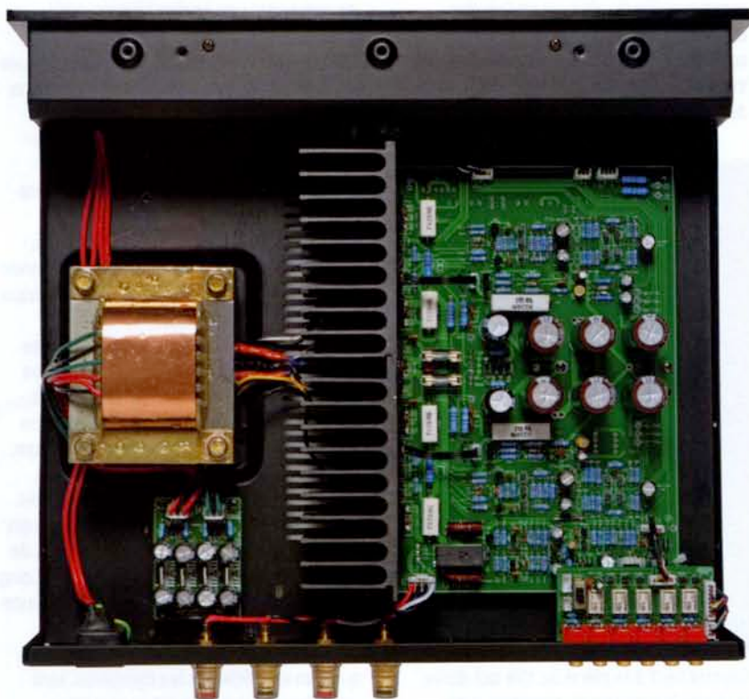
À gauche, le transformateur de 500 VA et ses circuits de régulation. À droite, la carte des amplificateurs ne comportant que des composants discrets.
